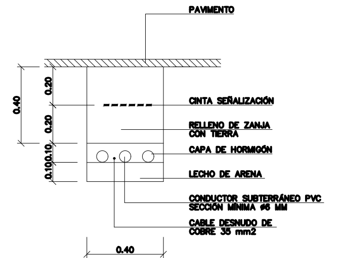
ZANJA DE ALUMBRADO PÚBLICO BAJO ACERADO
