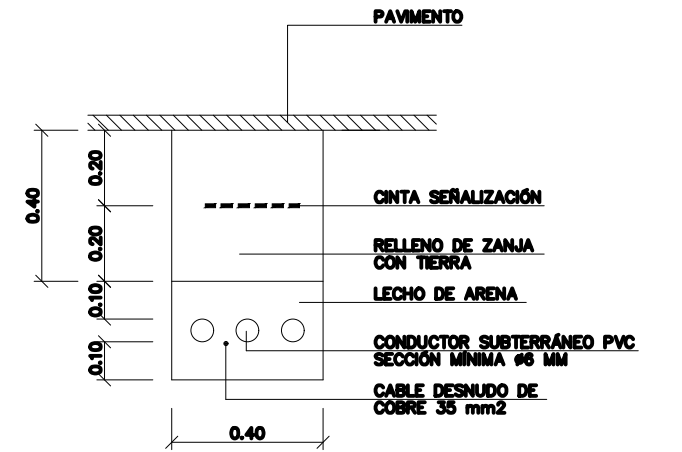
ZANJA DE ALUMBRADO PÚBLICO BAJO ACERADO
